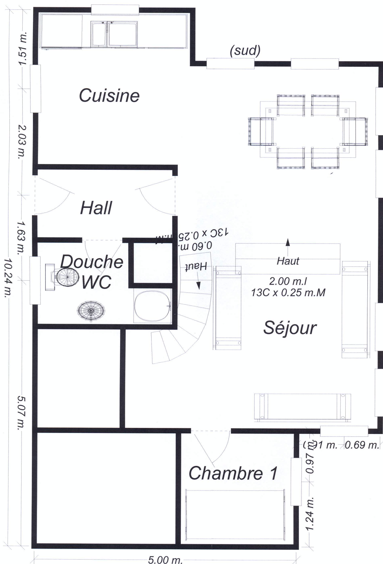
Chalet Casi Jappi (rez)
