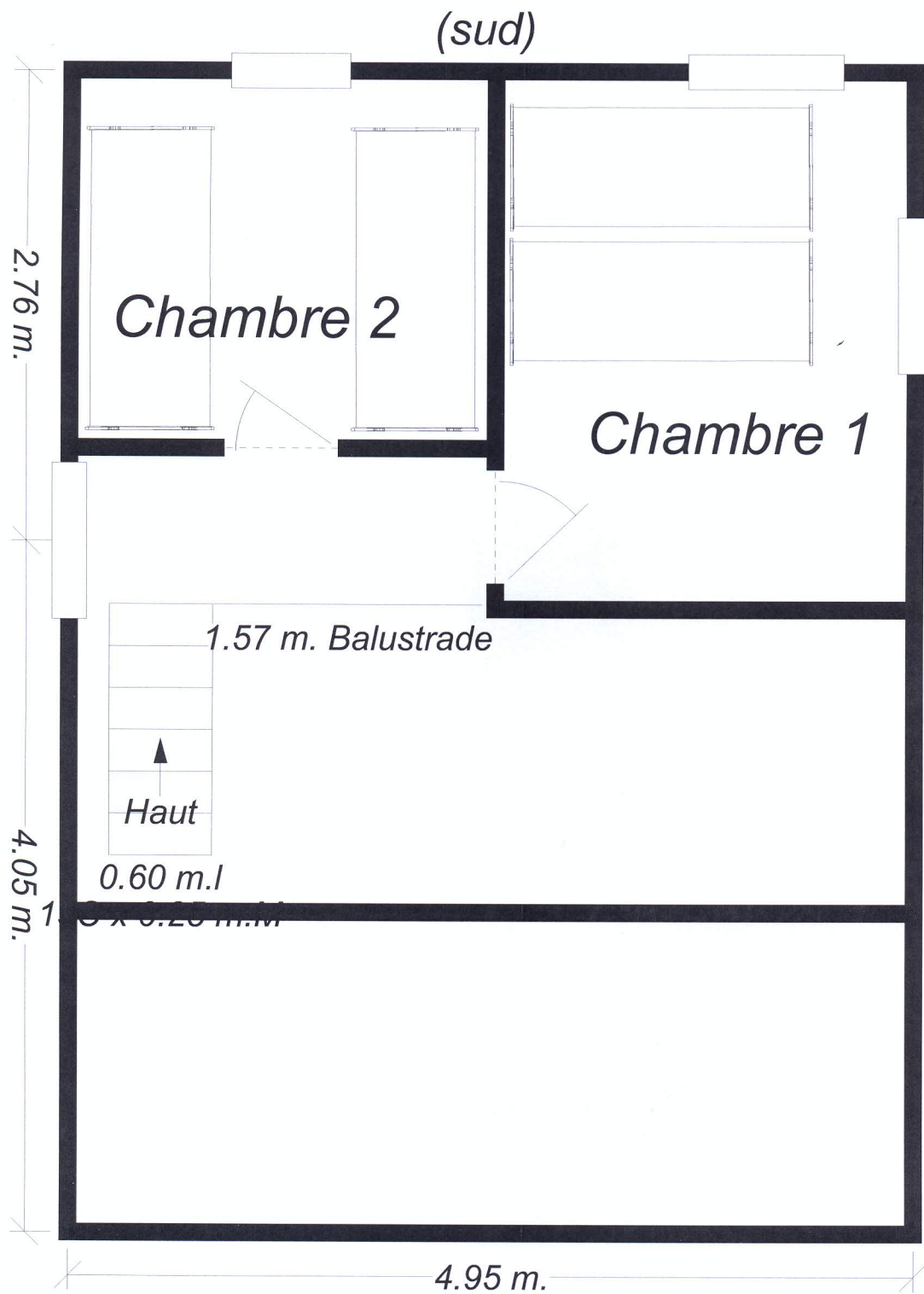
Chalet Pin d'Arolle (étage)
