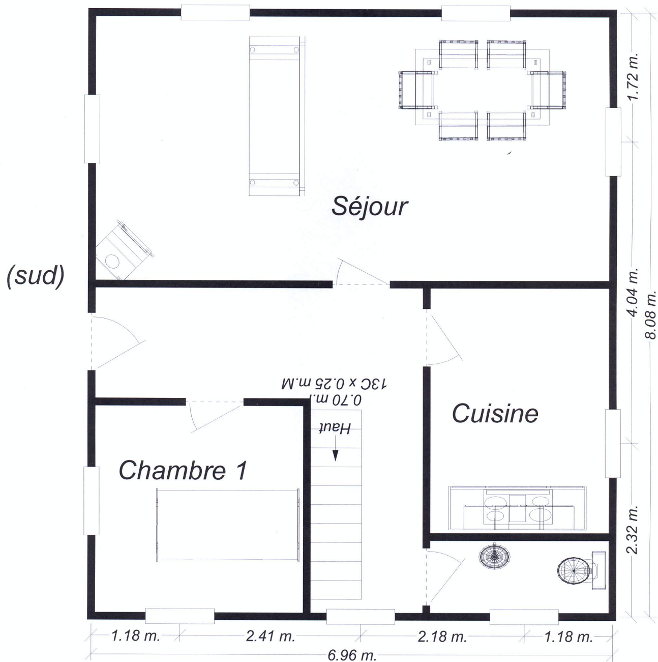
Chalet Pralonzet (rez)
