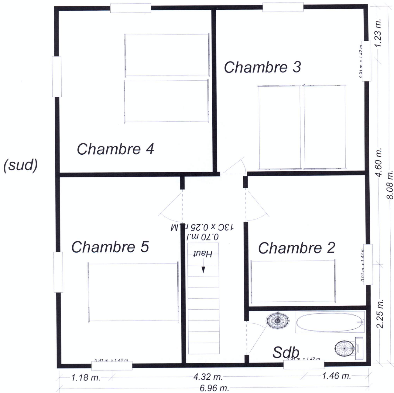
Chalet Pralonzet (étage)
